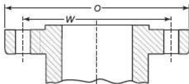
Flange
