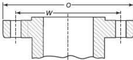
Flange
