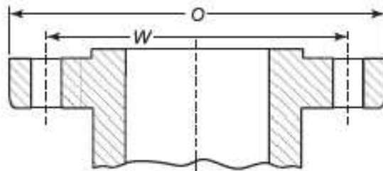
Flange
