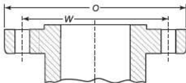
Flange
