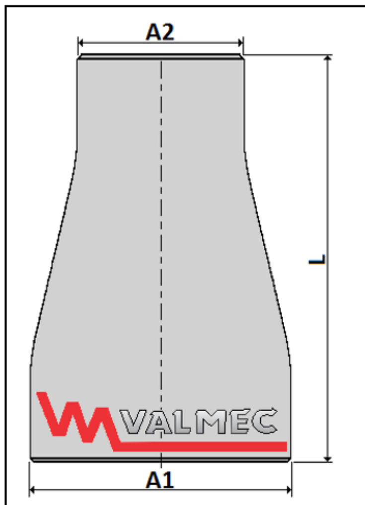
Dimensões conforme ANSI B 16.9;
