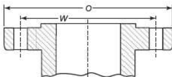
Flange
